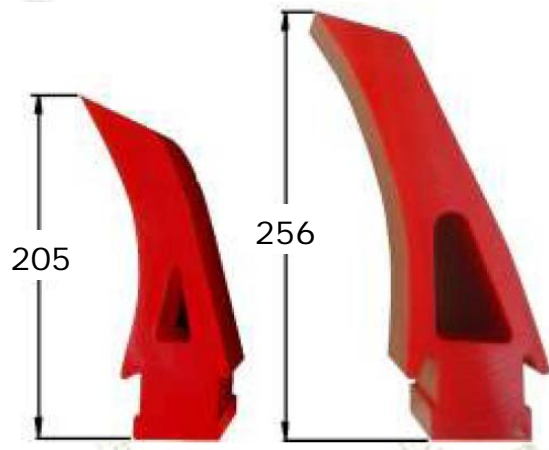
Normaal mes Bandsnelheid: ≤3.5m/s
