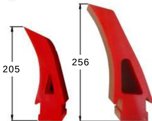
Couteau normal Vitesse bande \leq 3.5\text{ m/s}
