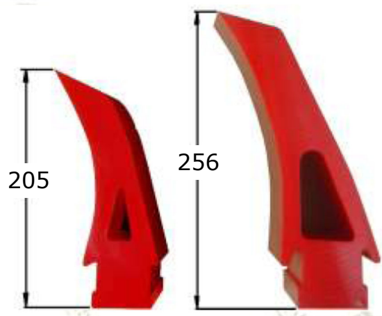
Normaal mes Bandsnelheid: \leq 3.5 m/s
